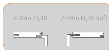
Priporočen podboj
