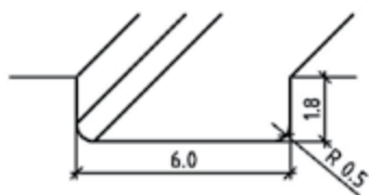
Detajl: vrezan motiv
